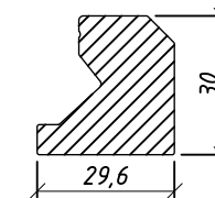
8-20/160 Leak Proof Gutter side-sealprofile Artikelnr. : 5448013 (L=250mm)
