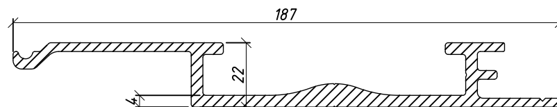
Alu 8/160 Leak Proof T subdeck (Slide-in) Artikelnr. : 871.5177
