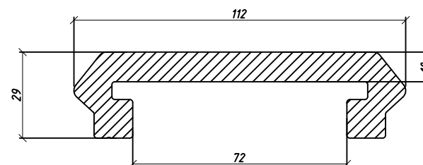
Aluminium endstop T-subdeck LP floor Artikelnr. : 5448006 L=350mm
