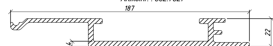
Alu 4/160, LR/LP, T-subdeck plane gutter area (slide-in) Artikelnr. : 862.7827
