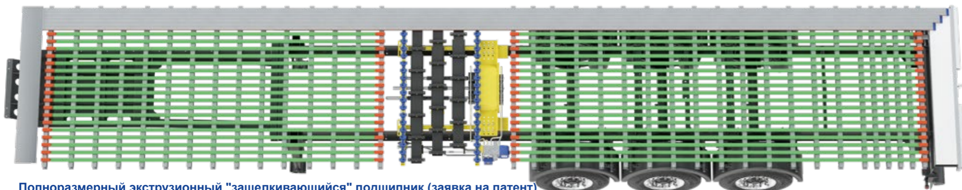
Полноразмерный экструзионный "защелкивающийся" подшипник (заявка на патент)
