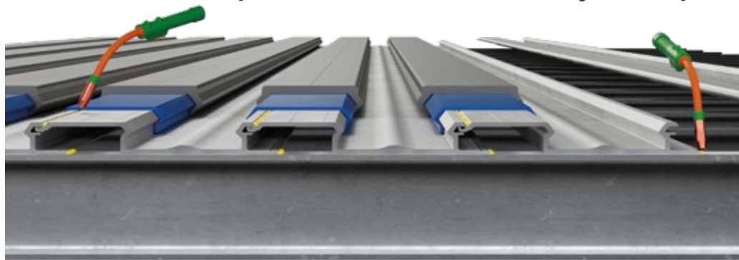
профили "Slide in", приваренные к алюминиевым поперечинам (в качестве альтернативы - клепаны), уплотненные сварными швами по всей длине.
