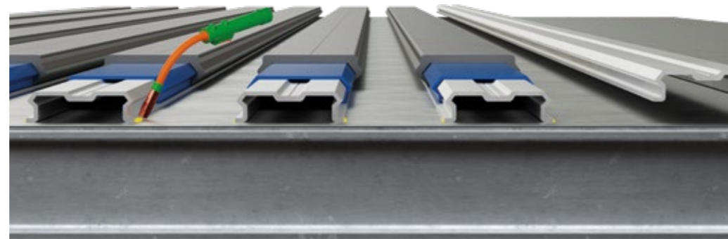
Свободные алюминиевые подпалубные профили, приваренные к алюминиевой гладкой пластине.
